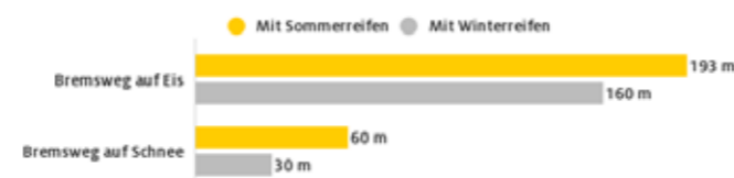
Bremsweg bei einer Geschwindigkeit von 50 km/h auf Eis und Schnee
