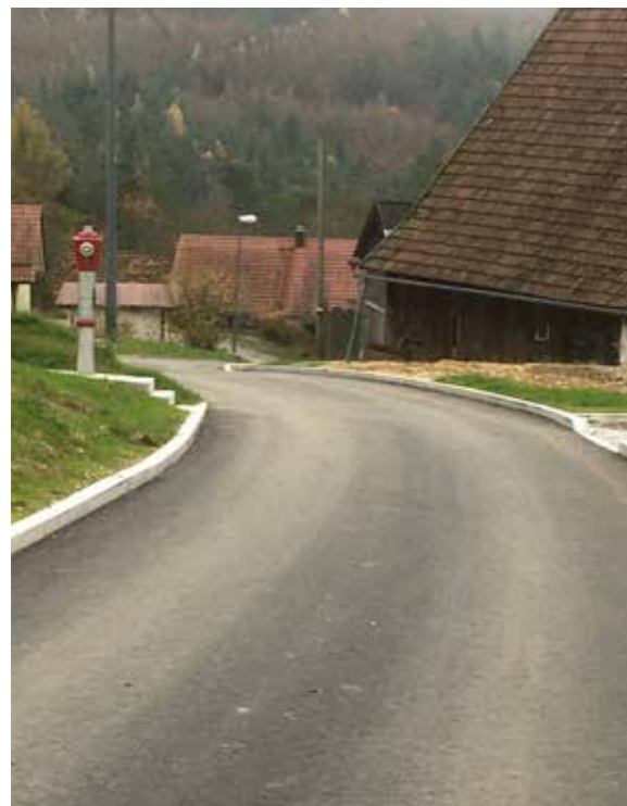
Vollausbau Heuweg: Gesamtbaulänge ca. 285 m Gesamtkosten: 201.000,-€ Förderung durch Amt für Ländliche Entwicklung mit 75% (incl. 10% ILE Bonus) Ebenso wurden bereits Speedpipes für den Glasfaseranschluß (FTTH) für 23.000,-€ mitverlegt.
